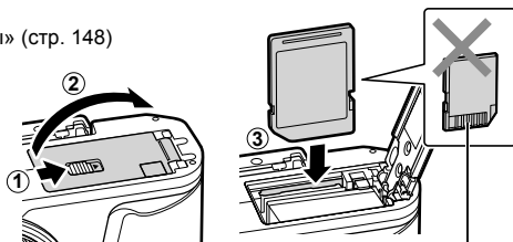
Расположение контактов
