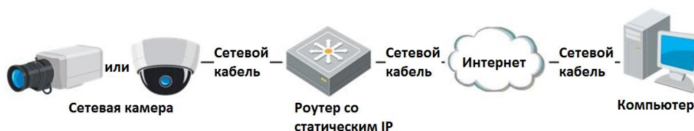
Рисунок 2-10 Доступ к видеокamере через роутер со статическим IP-адресом
